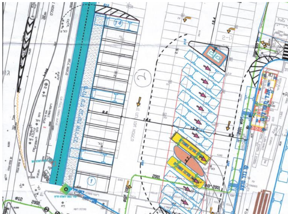
תרשים 3 – מיקום עמדת טעינה בין שני רציפי חניה
