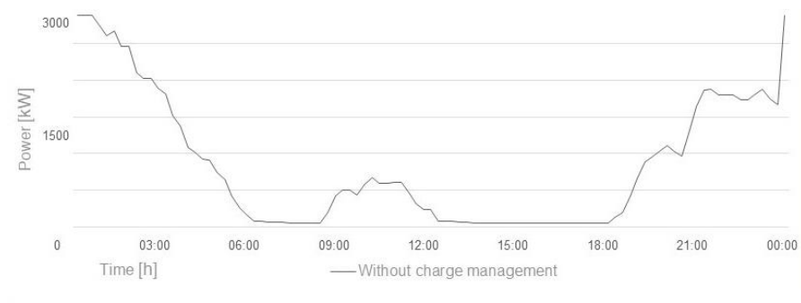
תרשים 1 – דוגמה לגרף צריכה יומי של מתקן תחבורה ציבורית
